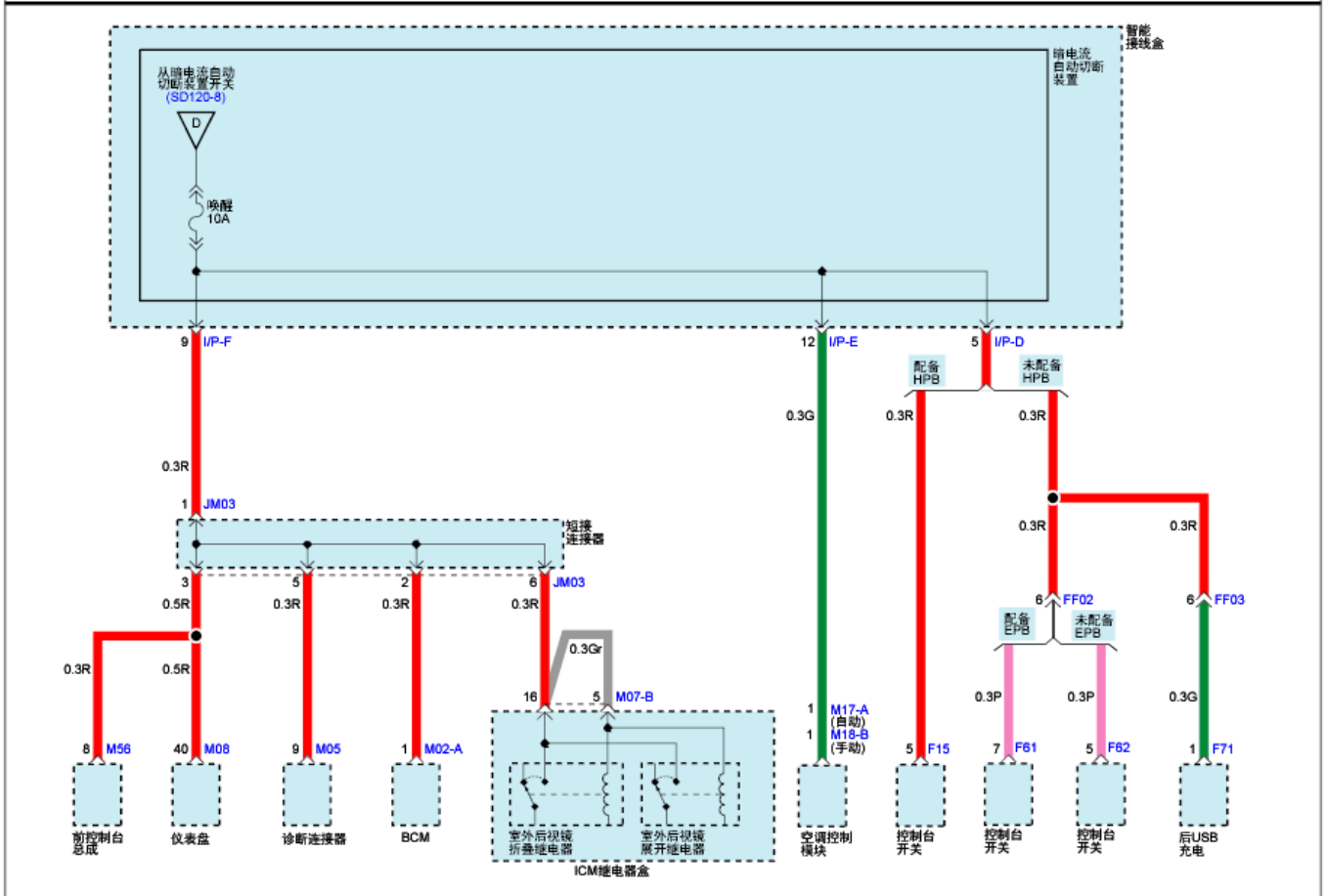
室内保险丝分布(9)
